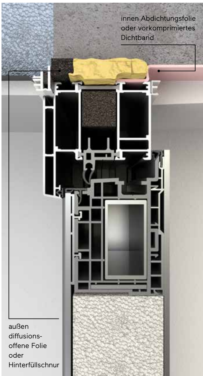
Einstufige Montage direkt auf Mauer
